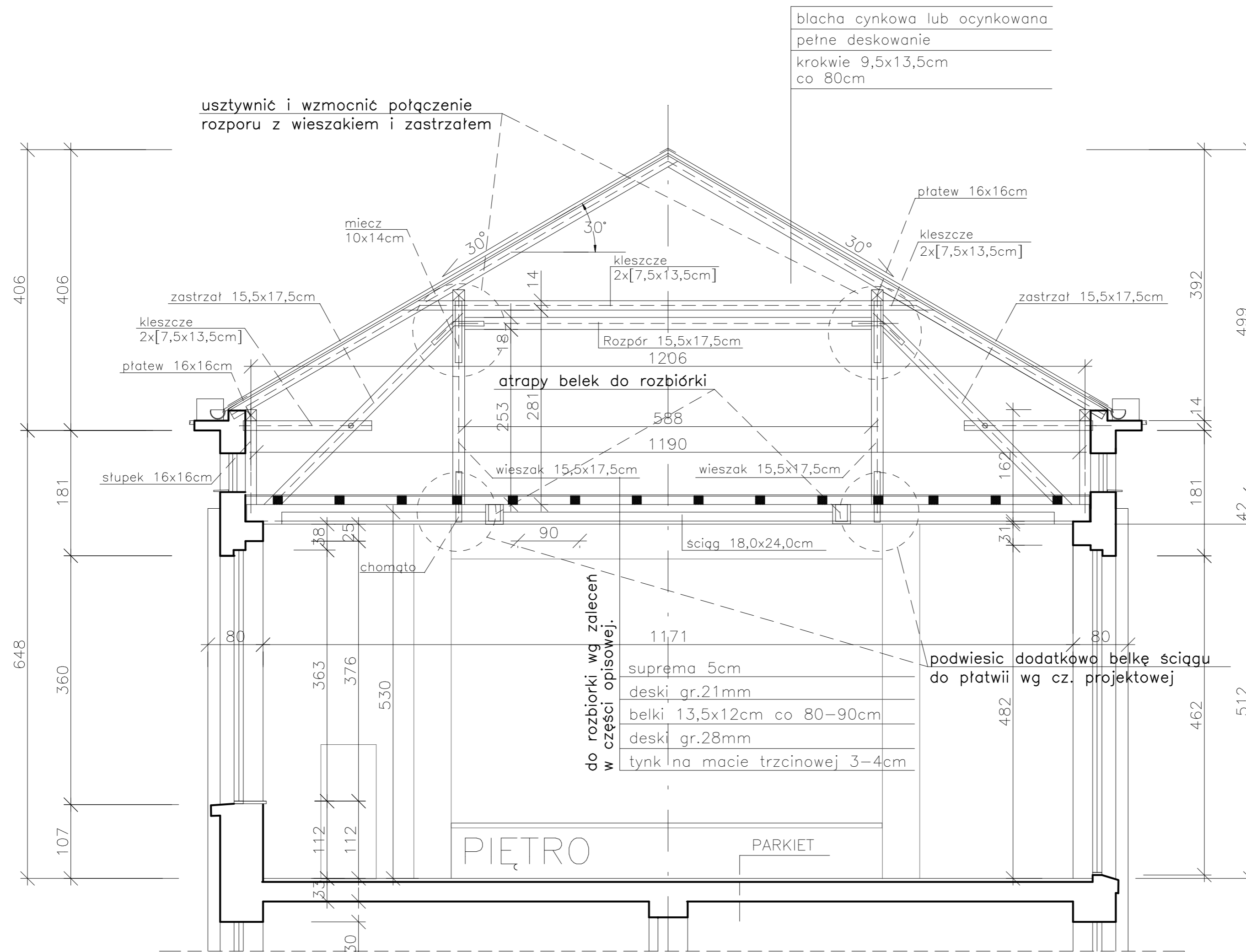
PRZEKRÓJ POPRZECZNY — 1:50
